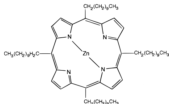
porphyrin 1
